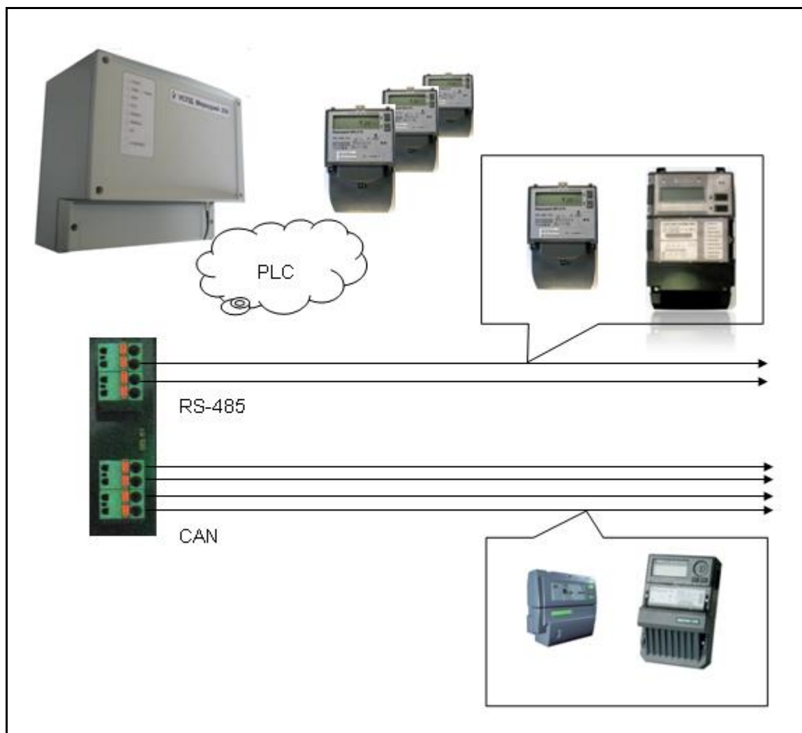
Рисунок Б.1 – Схема подключения УСПД
