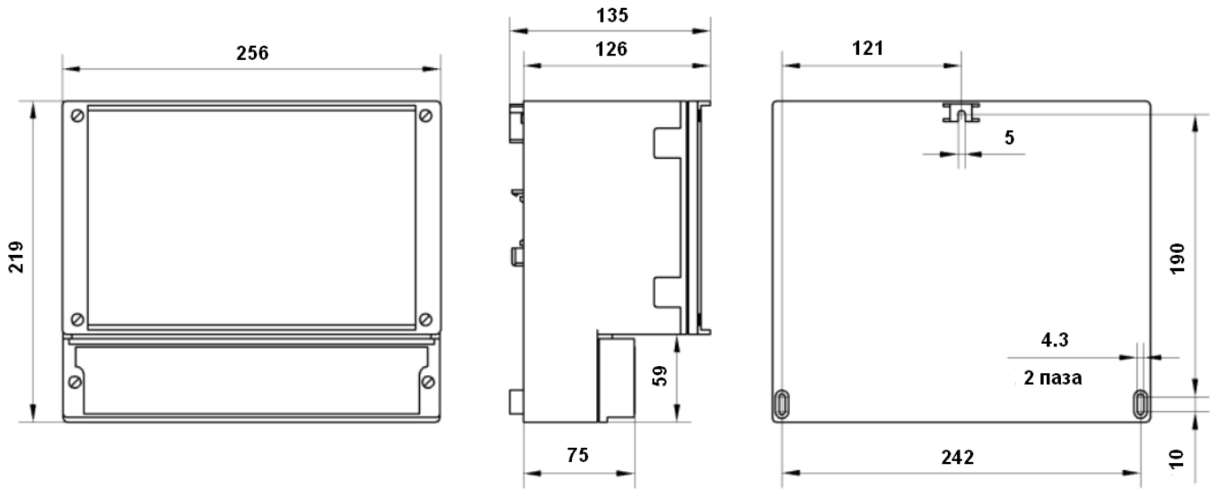
Рисунок А.1 – Габаритный чертеж УСПД
